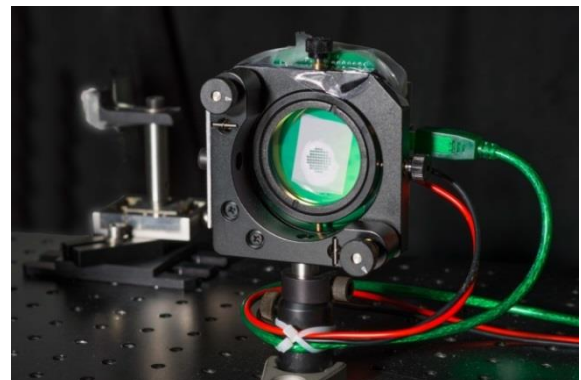
Prototype d'un miroir déformable thermiquement, installé sur la table optique principale de la plate-forme CALVA. © CNRS/Cyril Fréssillon
